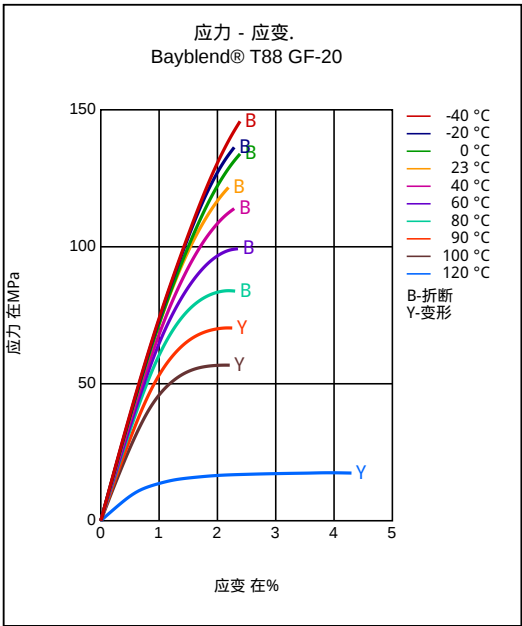
应力 - 应变.
